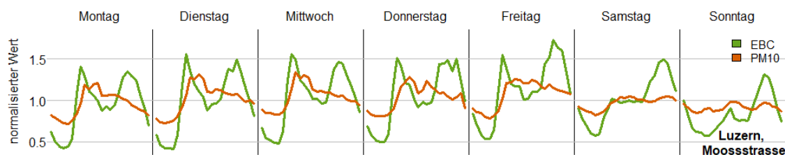
Abbildung 31: Wochengang der mit dem jeweiligen Jahresmittelwert normalisierten PM10- bzw. EBC-Werten des Jahres 2021 an der Messstation «Luzern, Moosstrasse».
