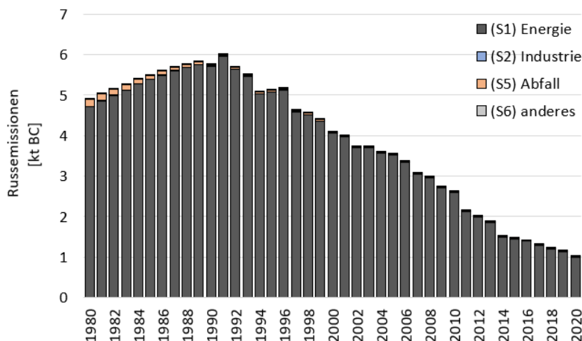
Abbildung 1: Russmissionen (BC) in der Schweiz nach Sektoren zwischen 1980 und 2020. 7
