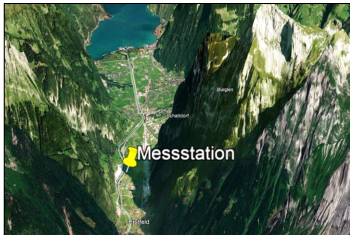
Abbildung 49: Die Messstation «Erstfeld, A2 Uri» in der topografischen Ansicht. Die Höhen sind um das Dreifache verstärkt. 55
