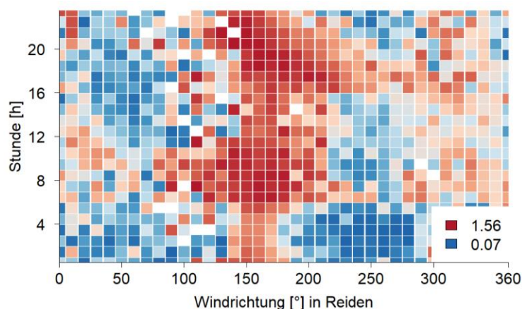
Abbildung 17: Windrichtungs- und Tagesganganalyse für die EBC-Messungen in Reiden im Jahr 2021.
