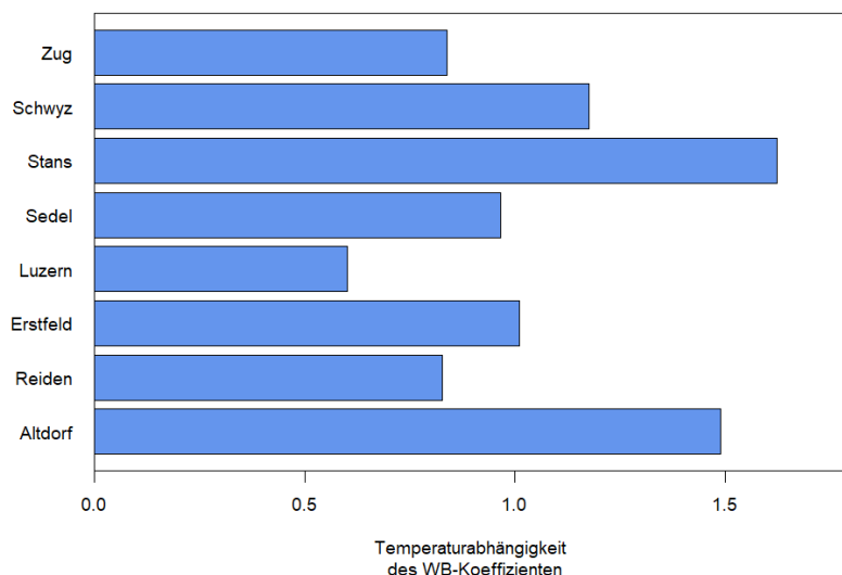
Abbildung 21: Temperaturabhängigkeit des WB-Koeffizienten aus dem Aethalometer-Modell, bzw. Betrag der Steigungen aus Abbildung 69 im Anhang. Zug und Schwyz zeigen Daten aus dem Jahr 2020, die anderen Messstationen aus 2021.
