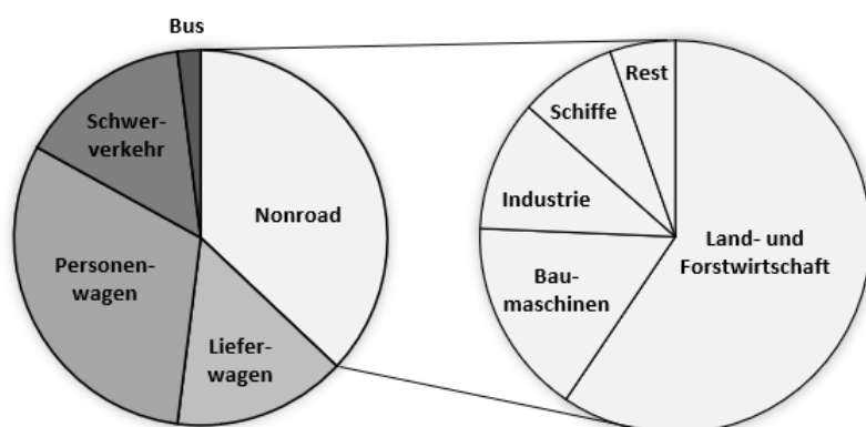
Abbildung 25: Anteile der Russemissionen von Dieselmotoren im Jahr 2010. 5
