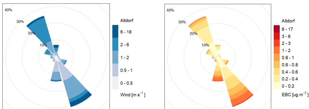
Abbildung 42: Wind- und Schadstoffrosen der Halbstundendaten des Jahres 2021 an der Messstation «Altdorf, Gartenmatt».
