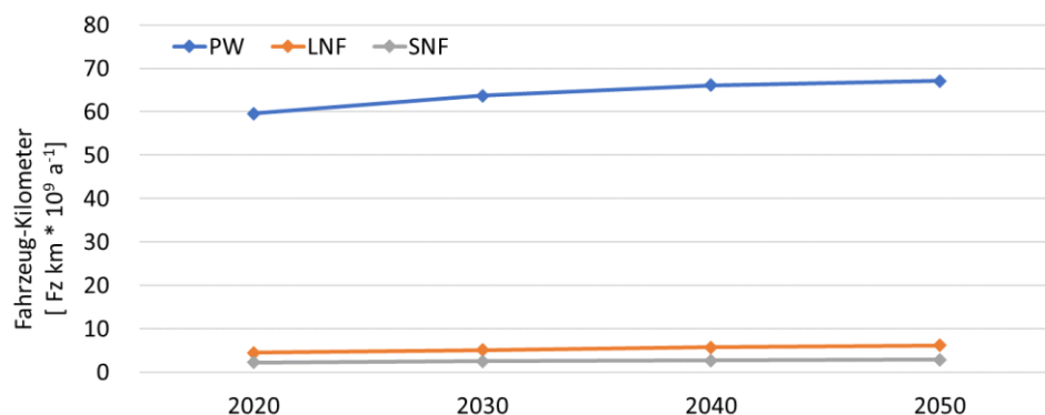
Abbildung 70: Entwicklung der Fahrzeugkilometer für Personenwagen (PW), leichte und schwere Nutzfahrzeuge (LNF und SNF) bis 2050 gemäss dem Bericht zu Energieperspektiven 2050+. 59
