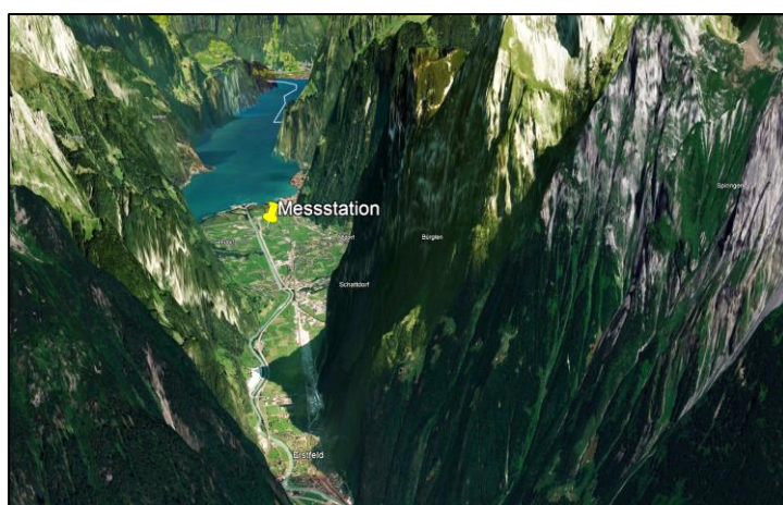
Abbildung 44: Die Messstation «Altdorf, Gartenmatt» in der topografischen Ansicht. Die Höhen sind um das Dreifache verstärkt. 54
