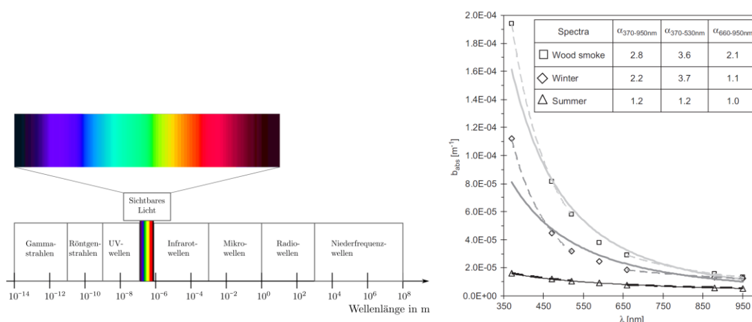
Abbildung 5: (a) Wellenlängen des Lichts mit dem ultravioletten Bereich ( \lambda = 100\text{--}380\text{ nm} ) und Infrarot ( \lambda = 780\text{--}1000\text{ nm} ), welche die physikalische Grundlage für das Aethalometer-Quellenmodell sind. 26 (b) Messungen eines Holzfeuers im Labor sowie Winter- und Sommerkampagnen in Roveredo zeigen, dass der Absorptionskoeffizient (« b_{\text{abs}} ») proportional zu « \lambda^{-\alpha} » ist, wobei « \lambda » die Wellenlänge und « \alpha » der Absorptionsexponent ist. Russ aus Verkehrsemissionen zeigen also eine schwache Wellenlängenabhängigkeit und somit ein tieferes « \alpha » als Holzfeuerungspartikel.
